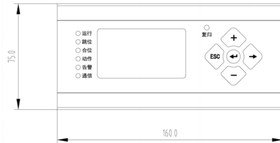
外形尺寸图
