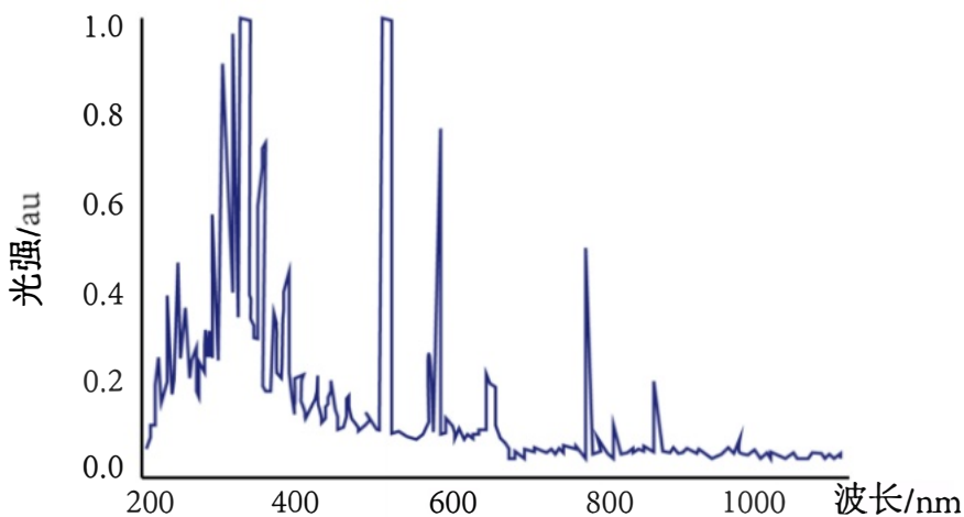
图三 铜电极电弧光光谱图
