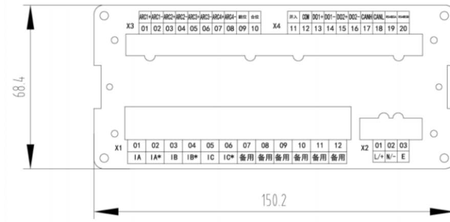
端子示意图
