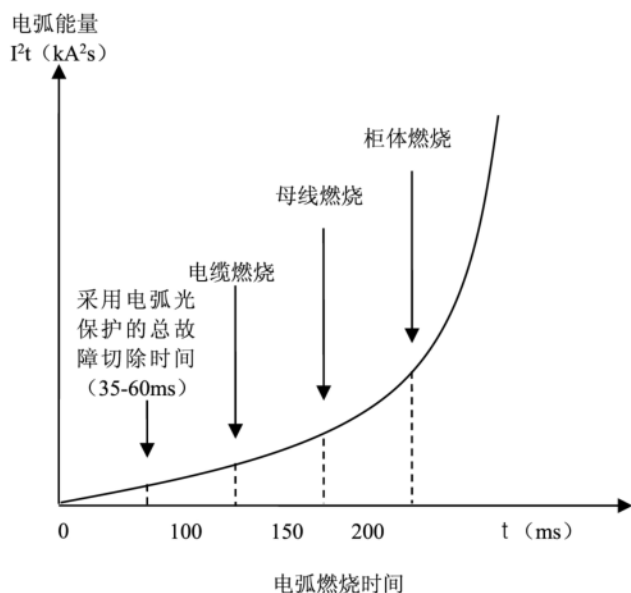
图一 电弧光的危害示意图
