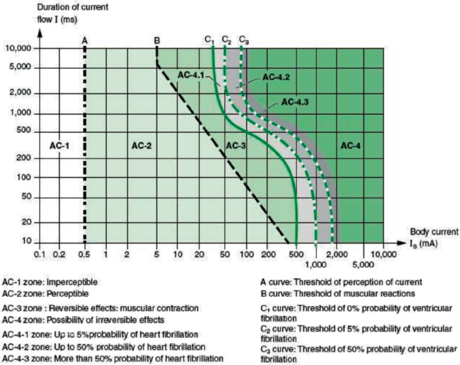
图四 IEC 经测试后得到的预期接触电压和允许最大通电时间之间的关系图
