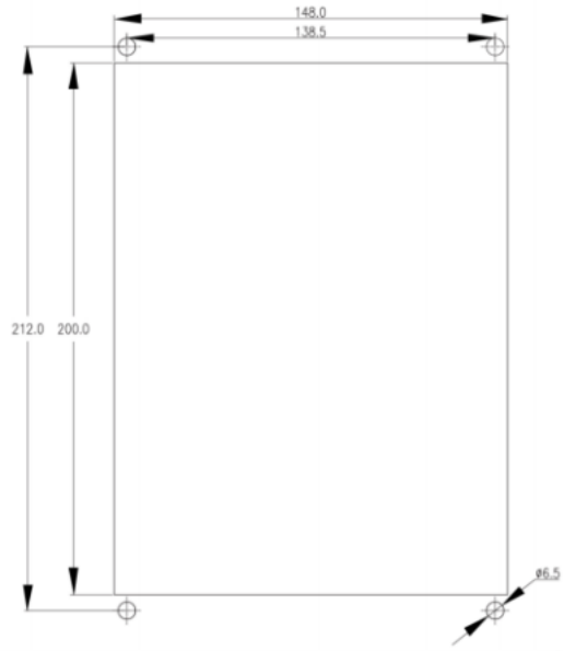
开孔尺寸图
